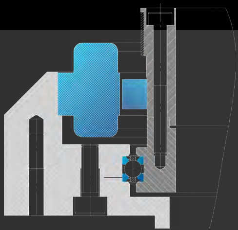
Konstruktionsbeispiel 1
