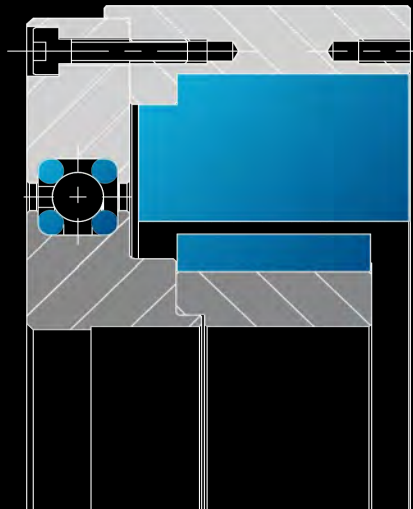
Speziallager mit Direktantrieb
