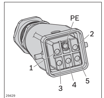
Anschlusskabelseite
